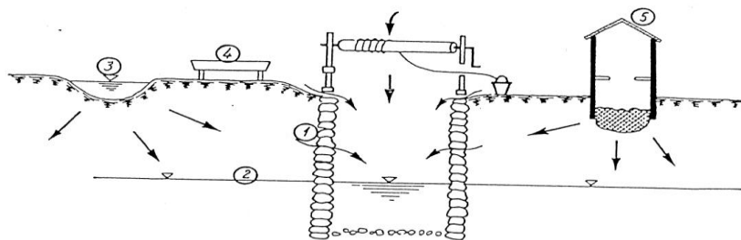
Nyitott, vedres, ásott kút szennyeződése
