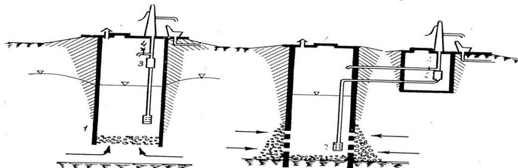
Zárt, ásott, szivattyús kút
